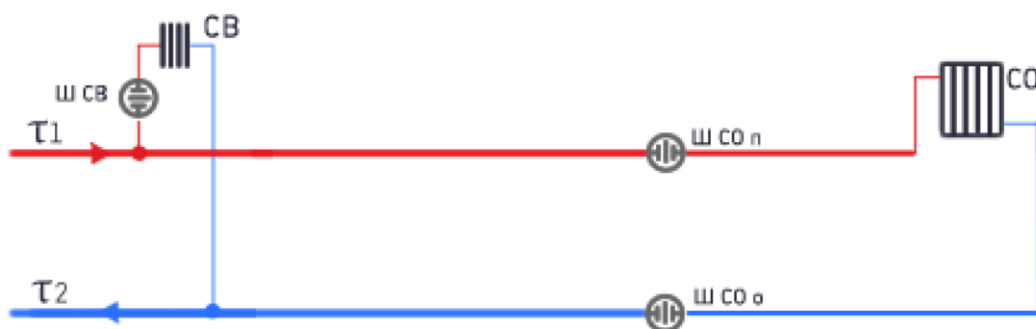
Рисунок 3 - Схема подключения потребителей к двухтрубной тепловой сети (при наличии внутренней системы отопления), зависимое присоединение, без смешения
