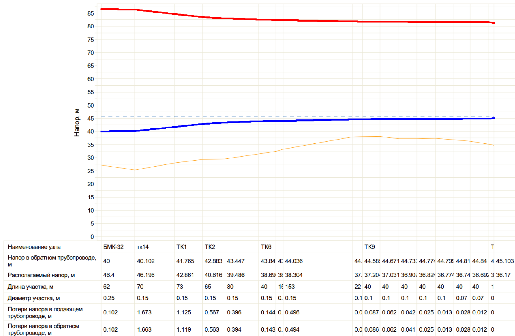
Рисунок 44 - Пьезометрический график от БМК-32 (с. Некрасовка) до определяющего потребителя – жилой дом (с. Некрасовка, ул. Парковая 13)
