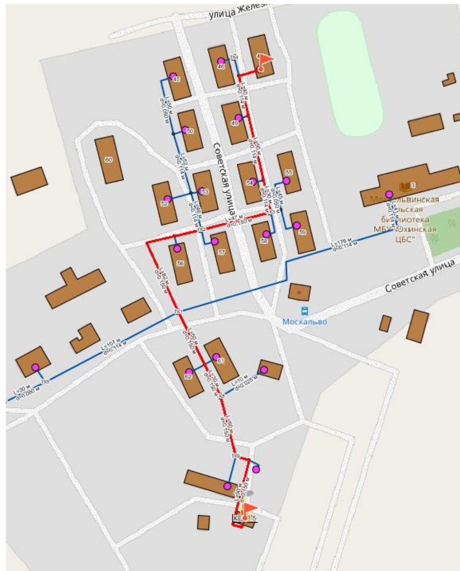
Рисунок 41 - Путь построения пьезометрического графика от Котельной КЕДР-5 п. Москальво) до определяющего потребителя – жилой дом (п. Москальво, ул. Советская 47)
